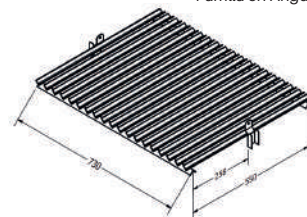
Parrilla en Ángulo V
