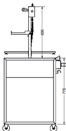
Vista Lateral Izquierdo
